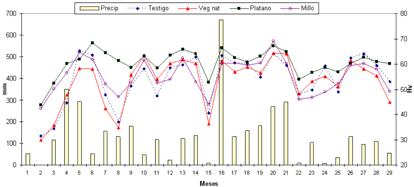
Figura 2: Comportamiento de la humedad del suelo con diferentes coberturas. Laboreo mínimo
