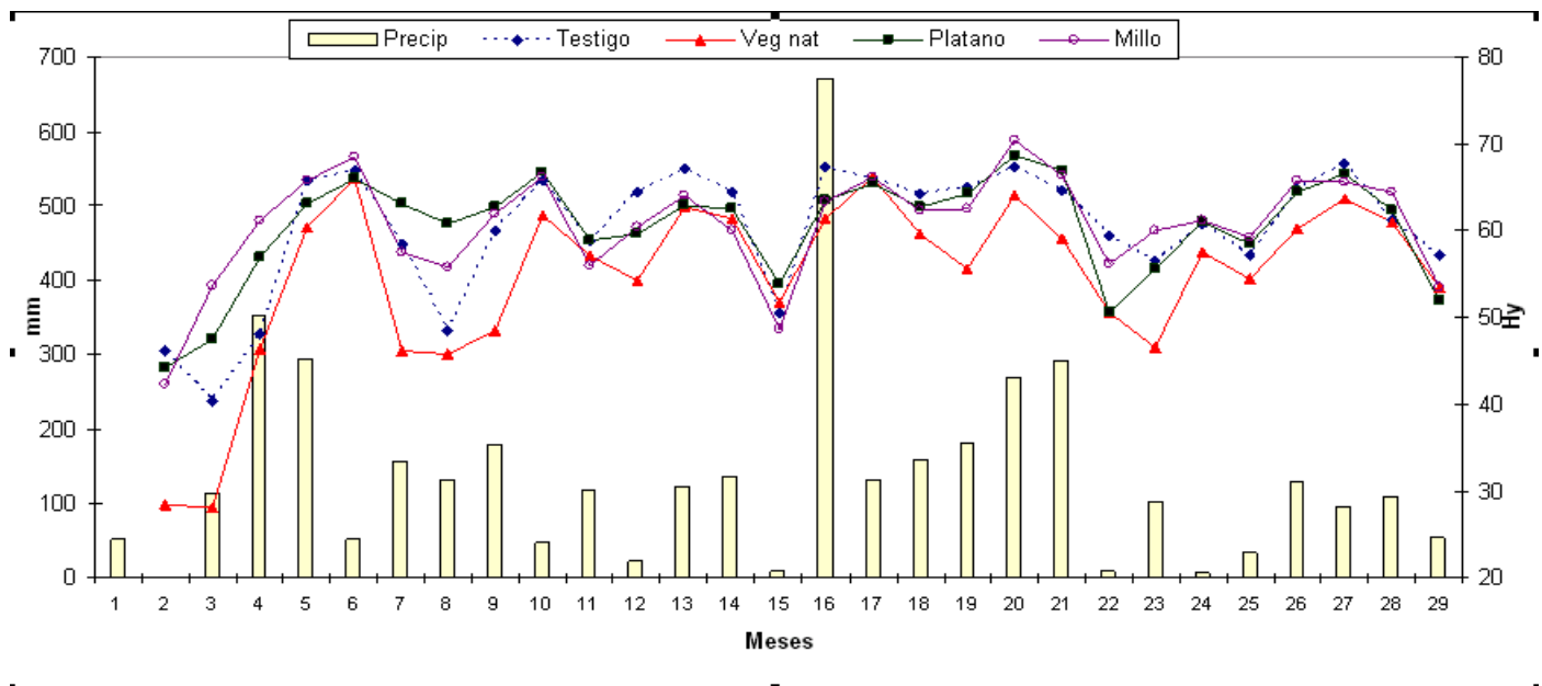
Figura 1: Comportamiento de la humedad del suelo con diferentes coberturas. Laboreo cero.
