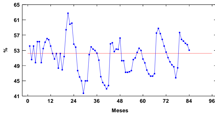
Fig. 1. Gráfica de serie de tiempo para eficiencia técnica de la inseminación artificial
