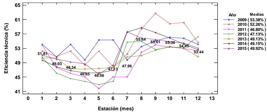
Fig. 5. Subseries anuales para la eficiencia técnica de la IA
