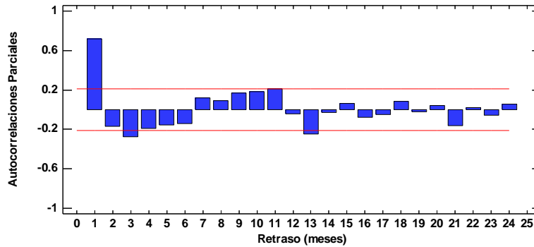
Fig. 2. Autocorrelaciones parciales estimadas para la eficiencia técnica de la inseminación artificial
