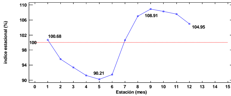
Fig. 4. Índices de estacionalidad para la eficiencia técnica de la inseminación artificial
