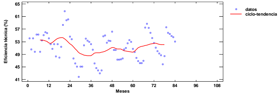
Fig. 3. Ciclo-tendencia observada para la eficiencia técnica de la inseminación artificial
