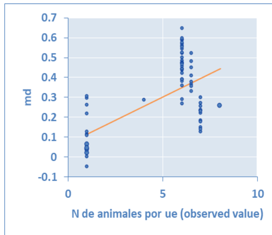
Fig. 3. Metaregresión análisis general: actividad GSH-Px en suero sanguíneo y número de animales por unidad experimental Coeficiente de regresión= 0,047 (P < 0,001)
