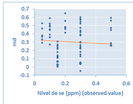
Fig. 5. Metaregresión análisis general: actividad GSH-Px en suero sanguíneo y nivel de selenio en la dieta Coeficiente de regresión= -0,1 (P = 0,002)
