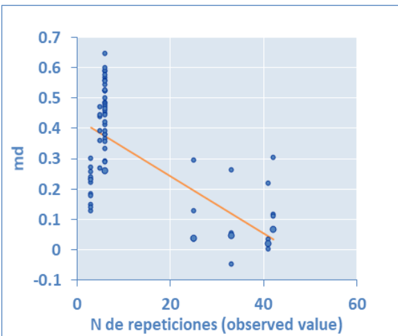
Fig. 2. Metaregresión análisis general: actividad GSH-Px en suero sanguíneo y número de repeticiones Coeficiente de regresión= -0,009 (P < 0,001)
