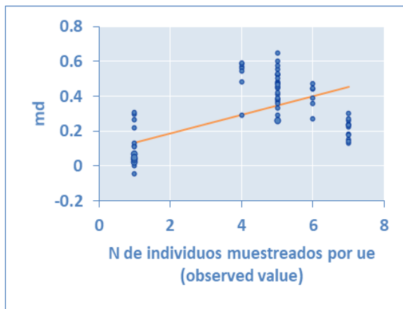
Fig. 4. Metaregresión análisis general: actividad GSH-Px en suero sanguíneo y número de individuos muestreados por unidad experimental Coeficiente de regresión= 0,053 (P < 0,001)
