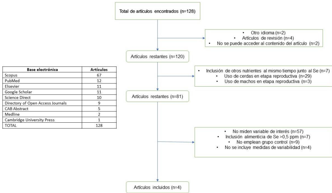
Fig. 1. Diagrama de flujo de exclusión y selección de artículos utilizados
